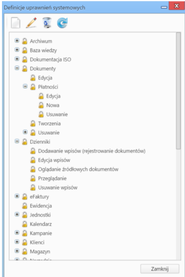
Drzewo uprawnień
