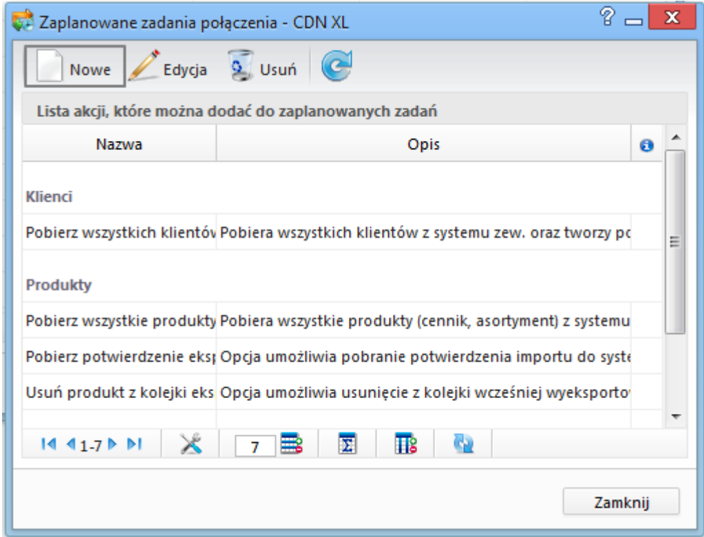
Rys. 13. Skonfigurowane akcje
