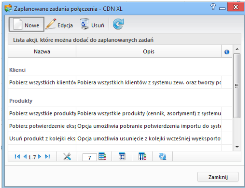
Rys. 13. Skonfigurowane akcje
